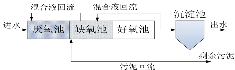
图 7-3 UTC 工艺流程图
