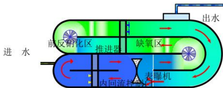
图 7-8 Carrousel 2000 型工艺原理
