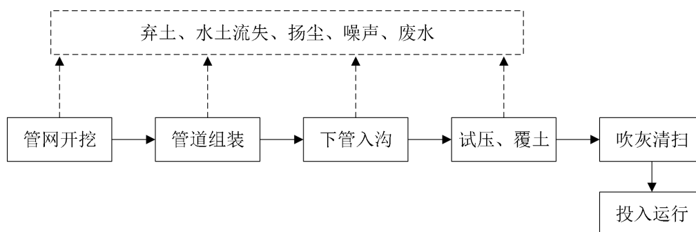
图 3-3 管道施工工艺流程及排污节点图
