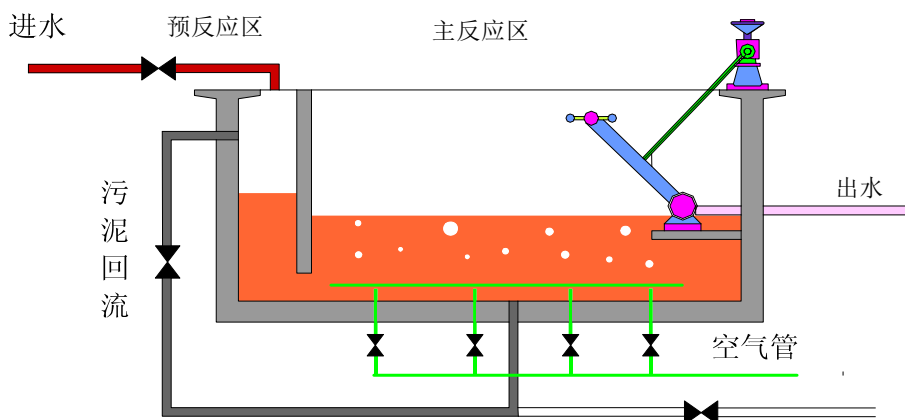
图 7-7 CASS 反应器基本构造
