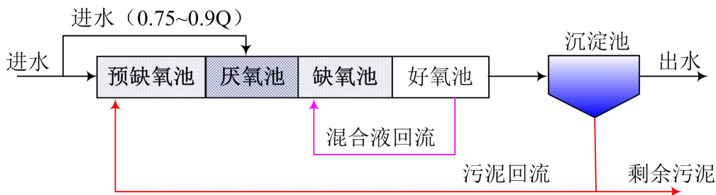
图 7-2 改良型 A 2 /O 工艺流程框图
