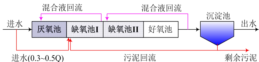
图 7-4 MUCT 工艺流程框图
