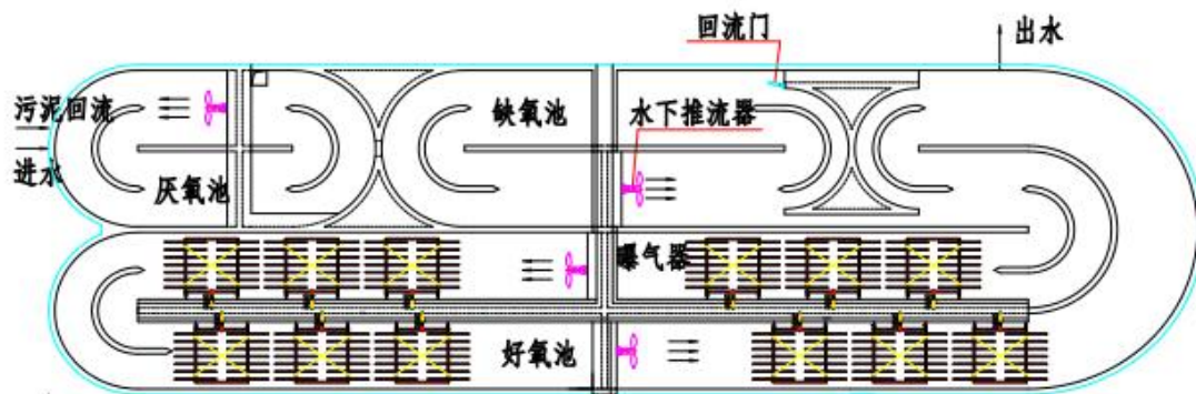
图 7-9 A/A/O 氧化沟系统原理图
