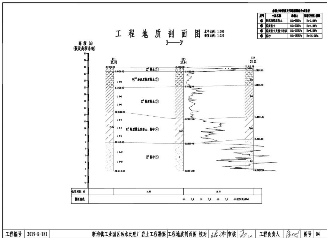
图 5-13 本项目场地工程地质剖面图（摘选）
