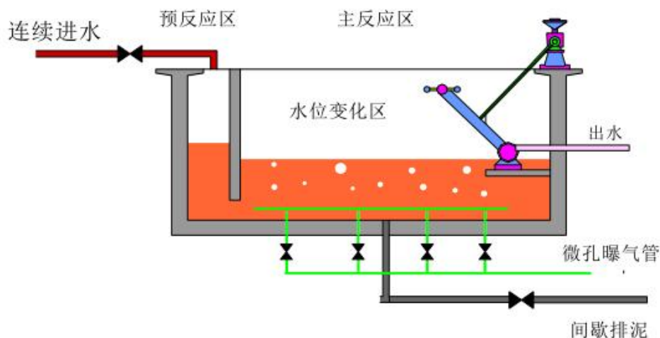
图 7-6 ICEAS 反应器基本构造
