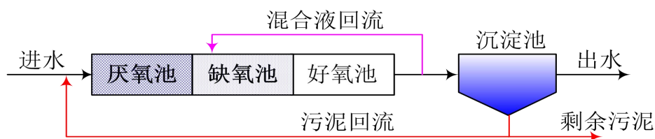
图 7-1 A 2 /O 工艺流程框图
