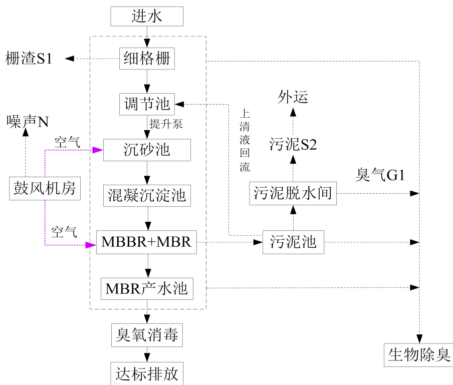
图 3-1 污水处理厂工艺流程及产污环节图
